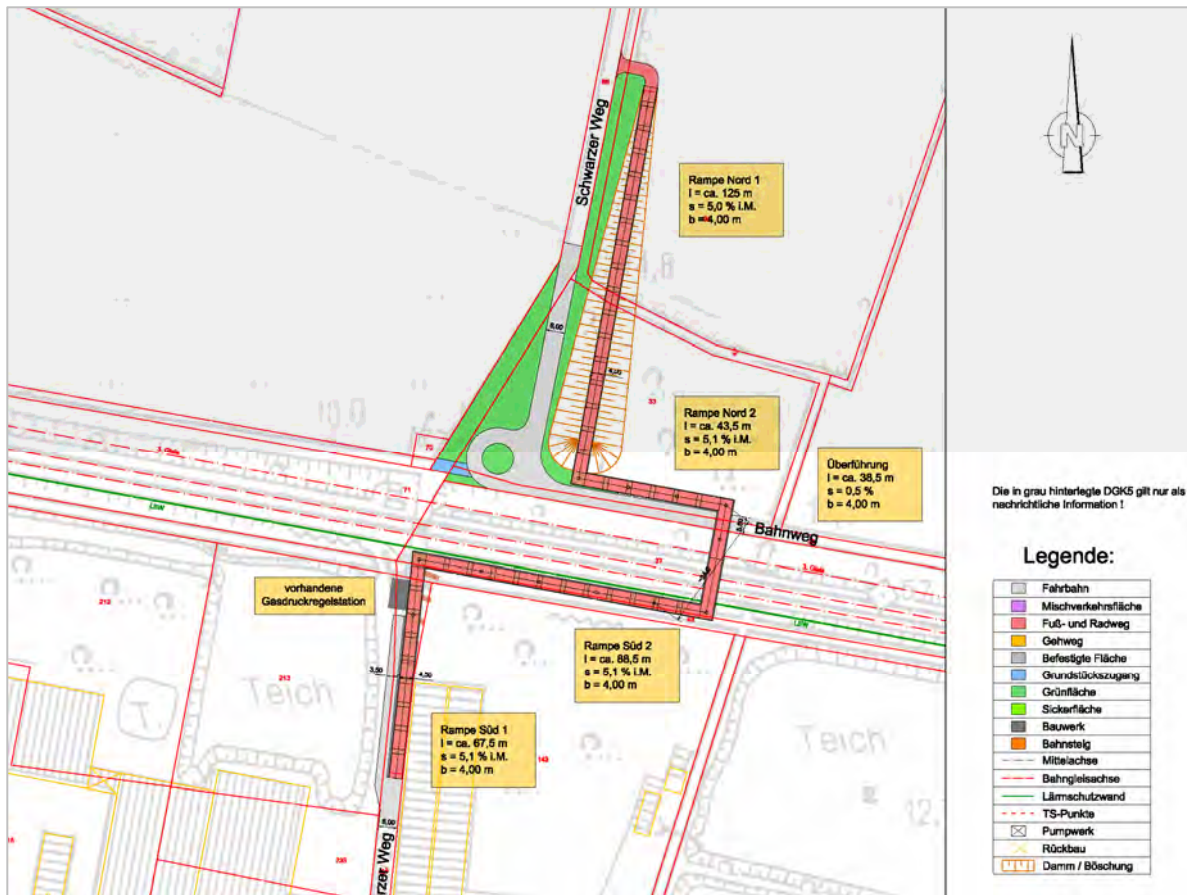
Vorschlag der Stadt Emmerich am Rhein (Ing.-Büro Spiekermann)
