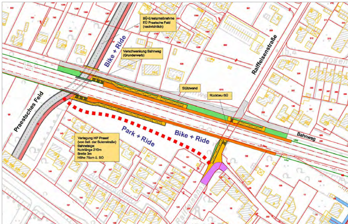
Systemskizze Bahnsteigverlegung (Ing.-Büro Spiekermann)
