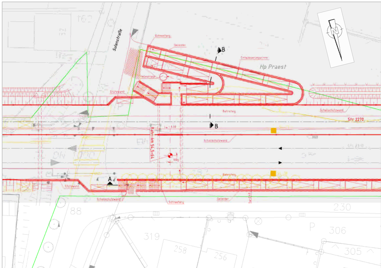
Auszug aus dem Bauwerksplan der DB AG (03/2010) – Bahnsteigverbindung
