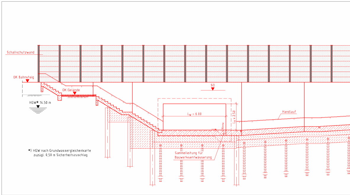
Schnitt A (unmaßstäblich) DB AG
